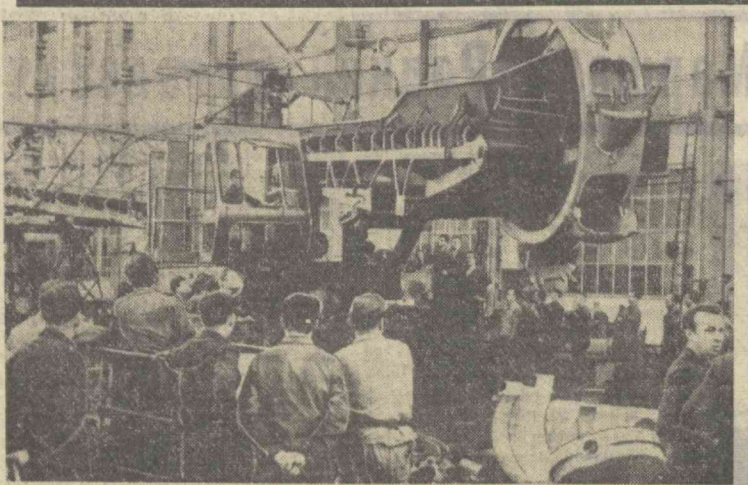
Бу роторли дизель экскаватор Лейпцигда очилган традицион баҳорги халқаро ярмақта Лауххаммере (ГДР)даги огир машинасозлик заводи томонидан намойиш қилинади. Катта ва кичик ҳажмидаги ишларни баъоринида куланиладиган ва агрегатнинг унумдорлиги соатига 500 кубометрди.
