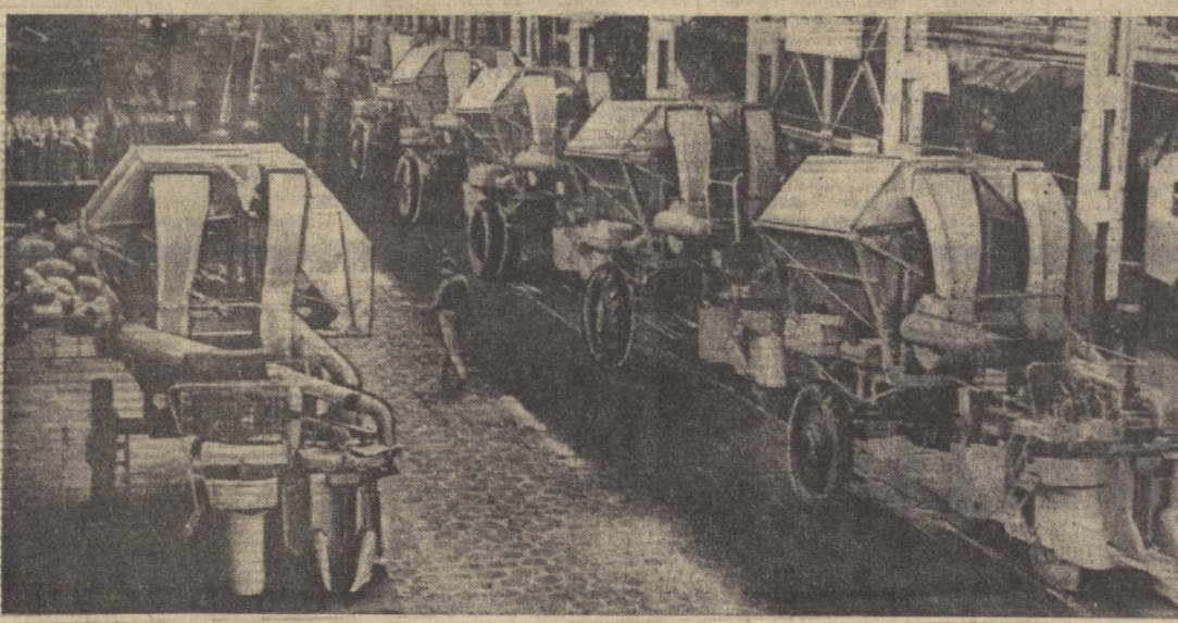
«Ташселмаш» заводининг ишчи ва мутахассислари муъ хосил ишдаида тер тўкиб ишлаётган пахтакорларимизга яна бир аjoyиб соғва армуғон эълдилар. Қорхона қонвейеридан тўрт қаторли пахта терим машиналари туша бошладилар. Бу янги серуни машина қорхона конструкторлари хамда пахтачилик машиналари бўнча Давлат махсус конструкторий бюроси ходимлари билан хамкорликда яратилган. Машинасозлар пахта йнгиим-терими бошлангунга қадар тўрт қаторли агрегатлардан 300 та таъбирлаб беришга аҳд қилганлар. Чапдаги суратда қорхонанин бош қонвейери 15-сехнини пешмадан йнгувчи леслари Ниша Зорова. Ундаги суратда эса янги машиналар учун барабанлар таъбирламокда.
