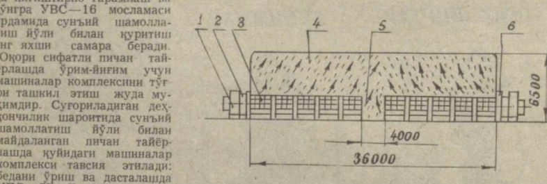
1-РАСМ. Икки вентиляцияли УВС—16 мосламасида пичан қуритиш схемаси. 1-вентилятор; 2-резент енг; 3-гарамлар остидаги канал; 4-гарам; 5-иссиқ узатгич; 6-изилоччи түсиқ.
