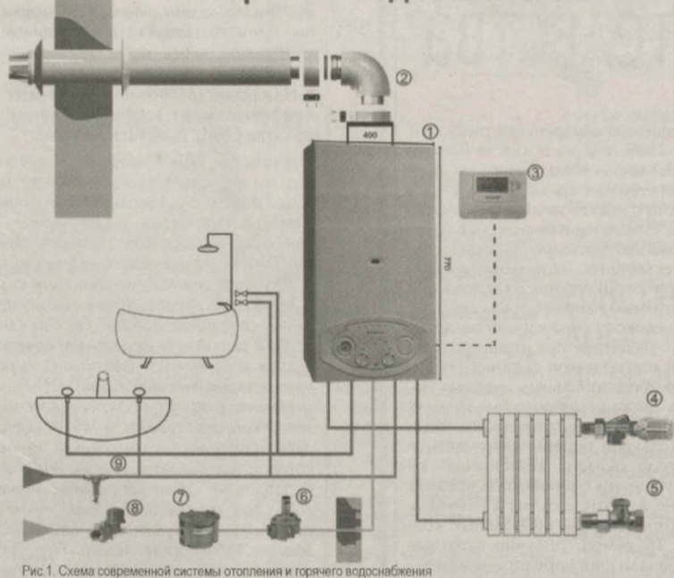
Рис. 1. Схема современной системы отопления и горячего водоснабжения
