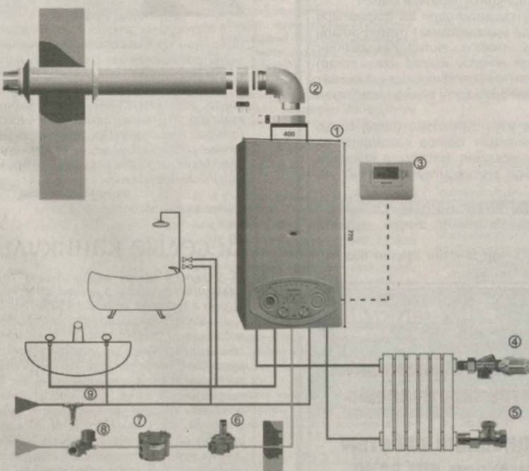
Рис. 1. Схема современной системы отопления и горячего водоснабжения
