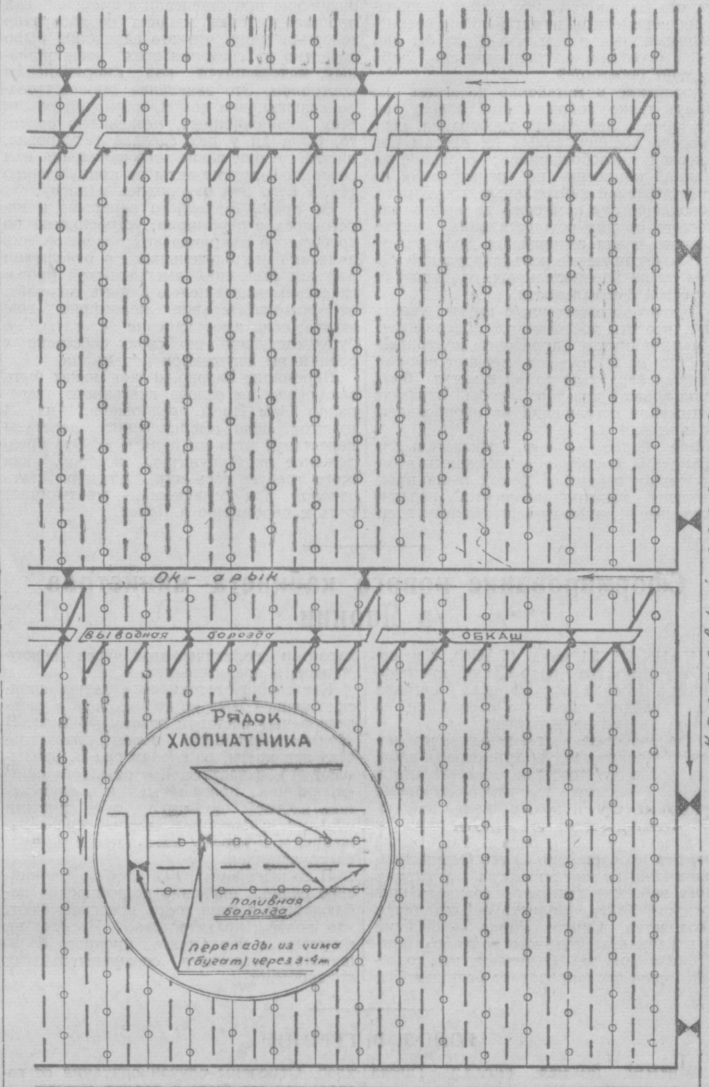
Схема регулирования поливной струи в бороздах на полях колхоза имени Молотова, Вуадильского района.
