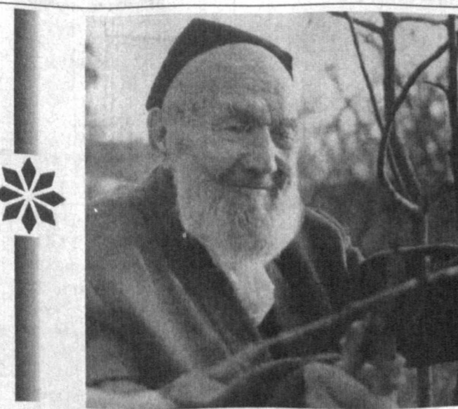
Эл аро «қариси бор ўйини париси бор», — деган нақб жорди. Мабодо Андижон томонларга йўналиш тушиб, Боғишмоқ даҳасида нақб сўз эста, «Янги ҳаёт» маҳалласида истиқомат қиладиган пир бадавлат отахон Абдурауф Аскарнинг сўбати олиш. Ана шунда бу ҳақимнинг аса мўҳаббини тоғандек бўласиз. 106 ёшли бу отахон тўрда доғали даврларни бошдан кечирган бўлса-да, аини пайтда жуда тетик —
