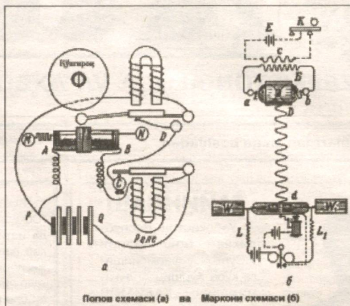
Попов схемаси (а) ва Маркони схемаси (б)
