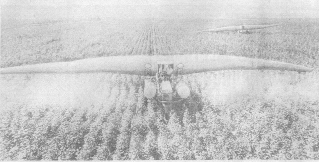
Как уже сообщалось в нашей газете, на полях совхоза имени 60-летия ВЛКСМ Большевосточного района проходит испытание новой пневмоустановки для дефолиации хлопчатника. Она создана совместно с московскими конструкторами. На снимке: новая установка на полях совхоза.
