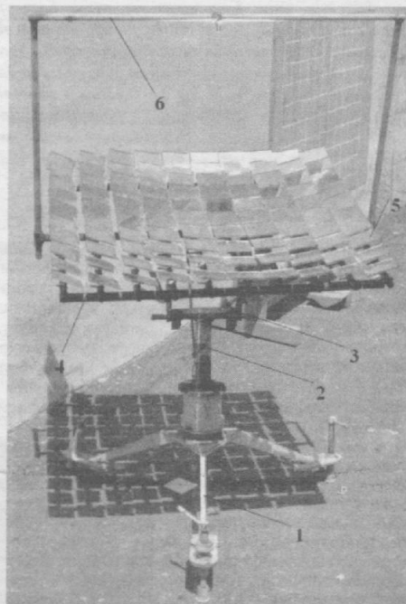
1-расм. «Куёш ошхонаси»нинг умумий кўриниши. 1-таянч, 2-вертикал айланиш ўқи, 3-горизонтал айланиш ўқи, 4-кўзгулар ўрнатиладиган каркас, 5-кўзгулар, 6-тутиқчи.
