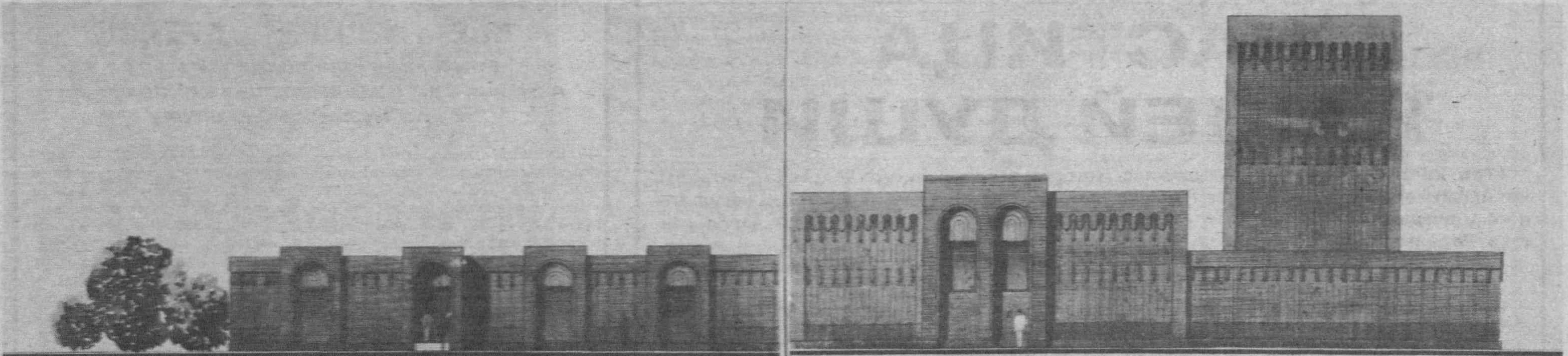
БЕКАБАДСКИЙ ХОКИМИЯТ. РЕКОНСТРУКЦИЯ ХОМИМИЯТНО ПОД ПЕРВОНАЧАЛЬНЫМ НАЗВАНИЕМ «ДОКА-ХЛЕБ» В П. БЕКАБАДЕ Ташкентская область. Проектное решение главного фасада
