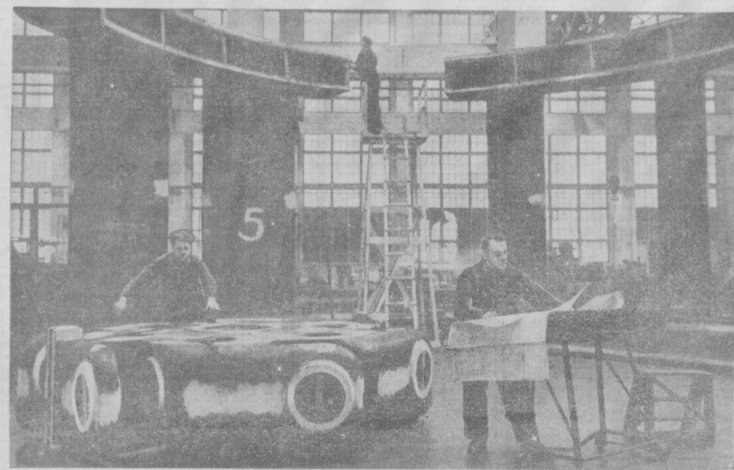
Ленинград. В гидротурбинном цехе металлического завода имени Сталина идет механическая обработка деталей турбины для Куйбышевской ГЭС. Над изготовлением этой сверхмощной машины трудятся лучшие рабочие — мастера турбостроения. На снимке: разметка статора и крошения турбины. На переднем плане — разметчик А. А. Дмитриев (справа) и С. А. Моторин, выполняющие за смену более двух норм. Фото П. Федотова. (Фотохроника ТАСС).
