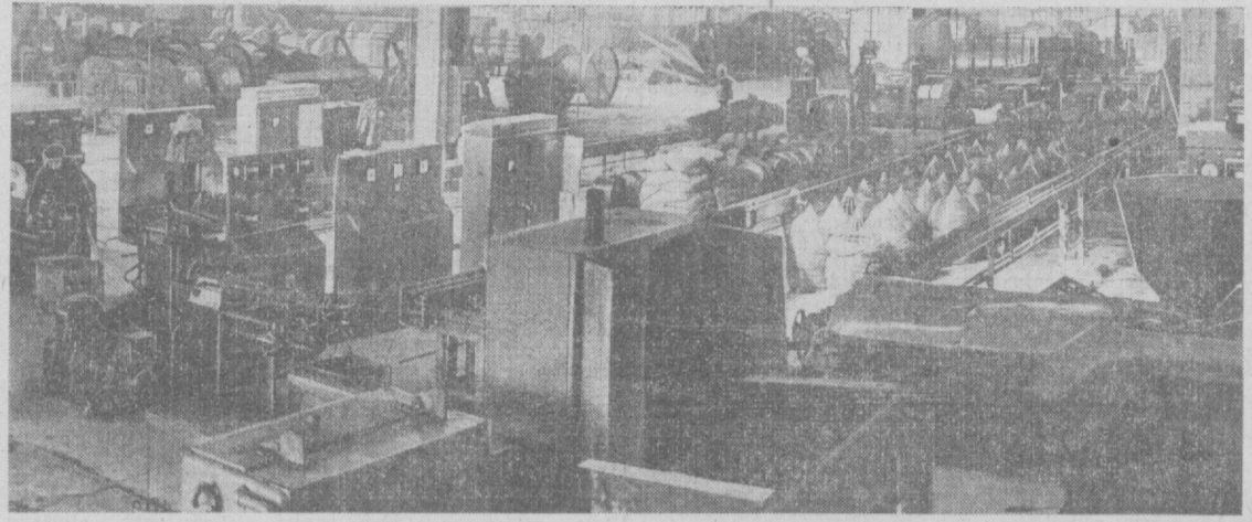
Так выглядит поточная автоматическая линия по производству жил телеграфно-блокировочных кабелей на заводе «Ташкабель».
