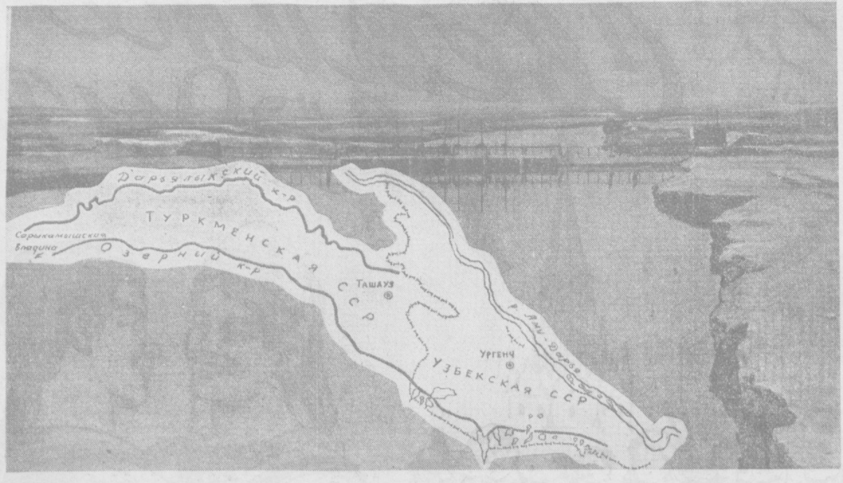
Схема Дарьяльского и Озерного коллекторов; вид на участок Озерного коллектора.
