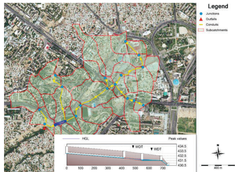
EPA Storm Water Management Model (SWMM) дастурий таъминотида subcatchment яратиш (Чорсу бозори мисолида).
