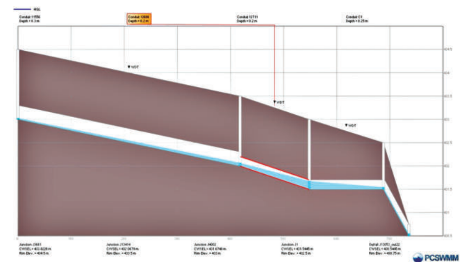
EPA Storm Water Management Model (SWMM) дастурий таъминотида ёмғир сувлари канализациясини моделлаштириш жараёнидан лавҳа (Чорсу бозори мисолида).
