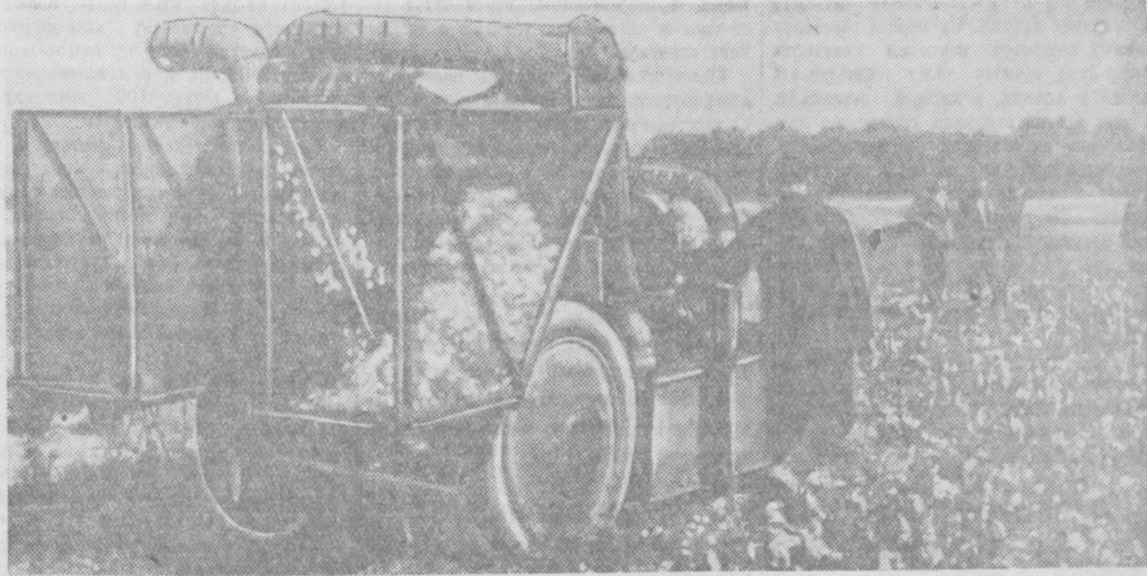
Испытание хлопкоуборочной машины на станции механизации СоюзНИХИ.
