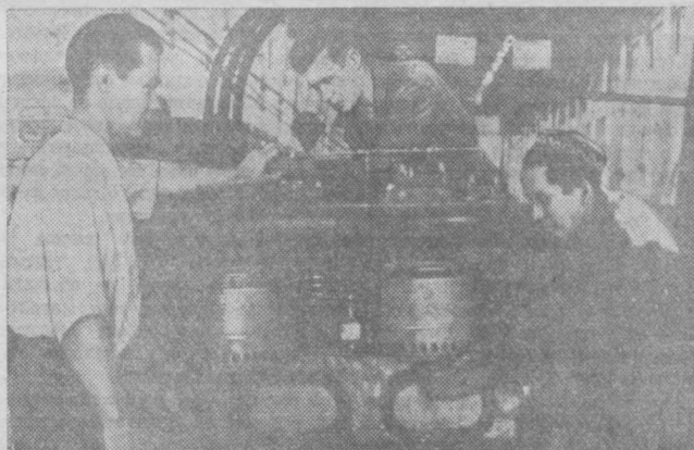
Ташкентский завод транспортного машиностроения освоил выпуск девятидюймовых компрессоров. На снимке (слева направо) начальник цеха В. Э. Гейдрих и слесари-сборщики Фахрид Худайбердыев и Насир Юнусов за сборкой компрессора. Фото В. Лейна.
