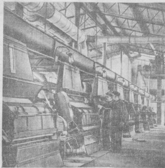
СУРХАН-ДАРЬИНСКАЯ ОБЛАСТЬ. К 1 Мая на Денауском хлопкозаводе вступил в строй действующих новый пухоочистительный цех. В нем установлены 22 пухоочистительные машины, которые будут ежедневно перерабатывать 220—230 тонн хлопка-сырца. НА СНИМКЕ: в новом цехе. Фото А. Кима. (Фотохроника УзТАГ).
