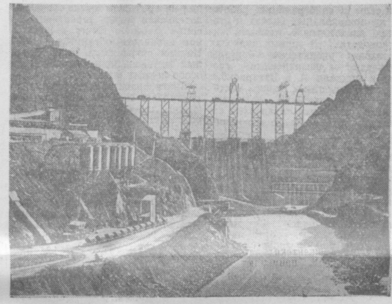
В штате Пенджаб (Индия) на реке Сабедри в 1946 году началось строительство комплекса сооружений энергетической системы Бхарна-Мангал. Это крупнейшая гидроэлектростанция Индии. Основным объектом системы является плотина Бхарна. Ее высота — более трехсот метров. В теле плотины расположены машинный зал электростанции, где будут установлены десять турбин мощностью по 90 тысяч киловатт каждая. Электростанция станции обеспечит нужды штата Пенджаб, а также будет передавать в Дели и в соседние штаты. В долине будет создано большое искусственное озеро, воды которого оросят почти полтора миллиона гектаров. НА СНИМКЕ: общий вид строящейся плотины Бхарна. Фото А. Ступина. (Фотокроника ТАСС).
