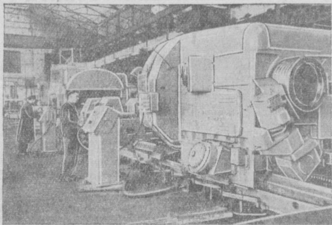
Ленинград. Завод имени Свердлова производит различные расточные станки высокого класса точности. Недавно в сборочном цехе закончен монтаж станка «ЛР-61»...
