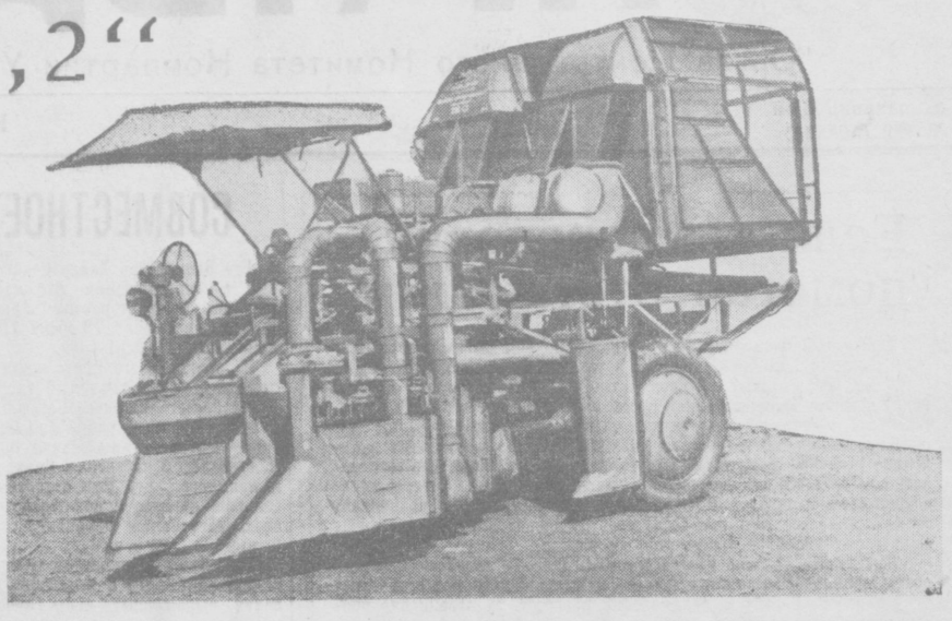
НА СНИМКЕ: хлопкоуборочная машина «ХВС-1,2».
