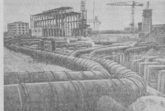
На строительстве Воронежской атомной электростанции. Сооружение главного корпуса. Фото А. Зенна. (Фотохроника ТАСС).
