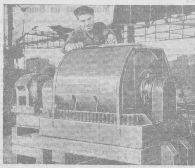
На ремонтно-механическом заводе Министерства промышленности строительных материалов УзССР изготовлена и опробована первая вибромельница...
