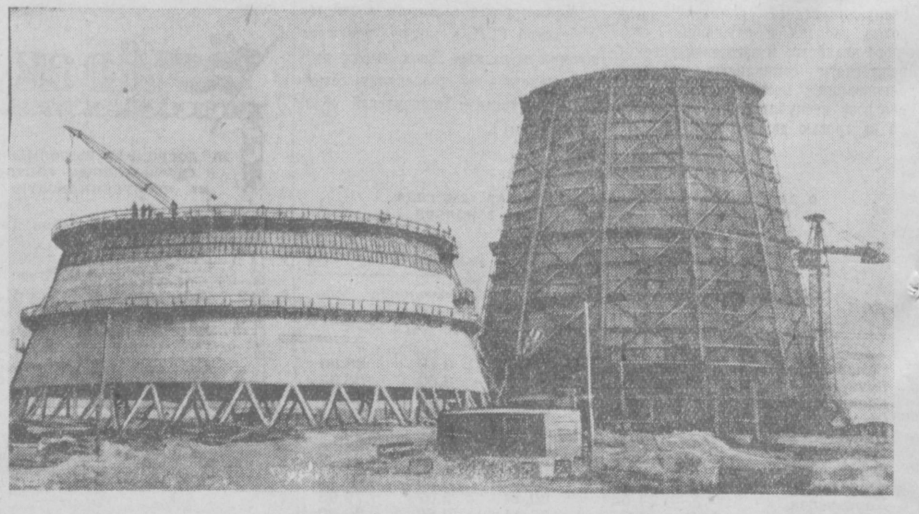
Для охлаждения воды Ангренской ГЭС строятся самые крупные в Средней Азии градирни с площадью охлаждения 1520 и 1600 квадратных метров и высотой 48 метров. Строители при сооружении градирен применили вместо обычных лесов подвесные металлические и сберегли этим государству 200 тысяч рублей. НА СНИМКЕ: общий вид строящихся градирен. Фото В. Лейзеровича. (Фотохроника УэТАФ).
