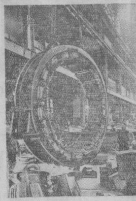
Ленинград. Коллектив завода «Электросила» имени С. М. Кирова в честь 40-й годовщины Великой Октябрьской социалистической революции объявил 7 ноября изготовить сверх плана два турбогенератора мощностью 100 и 50 тысяч киловатт, 10 крупных машин разных типов и различную аппаратуру. На снимке: работы по сборке электрогенератора. (Фотохроника ТАСС).
