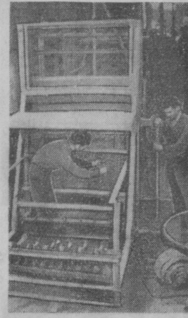
Новые прессы для производства камышитовых плит начал выпускать завод местной промышленности имени В. П. Чкалова. Первая партия этих машин уже отгружена колхозам, осваивающим новые земли в Голодной степи. На снимке: сборка новых прессов.
