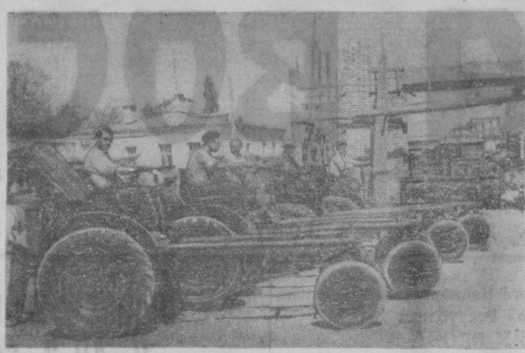
Тюрк-Курганская МТС непрерывно оснащается новой техникой. На днях поступили новые тракторные самоходные шасси марки «ДСШ-14», выпускаемые Харьковским тракторным заводом. С набором соответствующих навесных орудий эти машины могут проводить культивацию посевов с одновременным внесением в почву органико-минеральных удобрений. На снимке: новые самоходные шасси в Тюрк-Курганской МТС. Фото Е. Корниенко. (Фотохроника УэТАГ).
