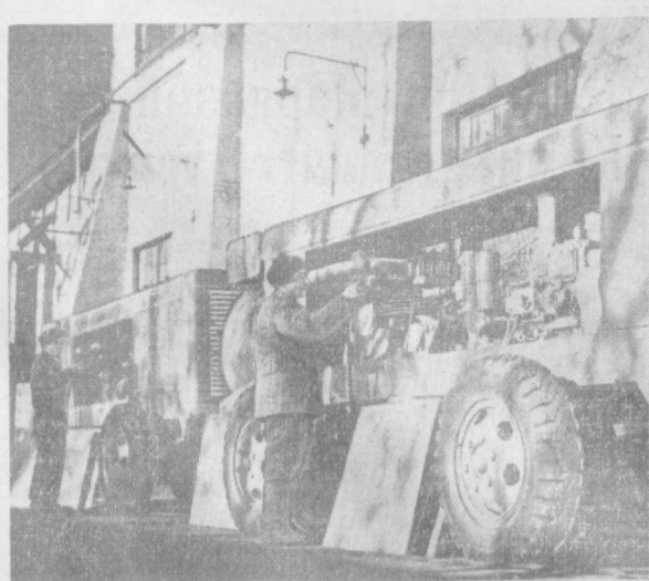
Тошкентдаги транспорт машиносозлиги заводи коллективига Кубага юбориш учун 40 та компрессор станцияси тайёрлаб вазифаси юклатилган эди. Коллектив бу фахрли заказни мудатидан илгари бажаришга қарор қилди. Суратда: Кубага юбориладиган «КС-9» компрессор станциясининг бўяш.
