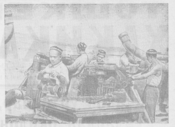
«Социализм» совхозининг 3-бўлим ишчилари пахта тани машинада теримга пахта тайёрлаган кўрмоқдалар. Бўлимдаги мажбур 9 та СХМ-48 пахта терим машинасини ремонтдан чиқаришди. Суратда: сўниги агрегатлар ремонт қилинмоқда. М. Шевелов фотоси.
