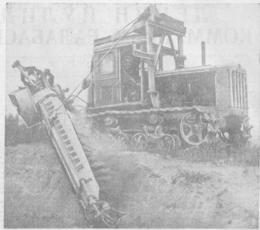
ТОШКЕНТ. Ирригация бўйича давлат махсус конструкторлик бюросининг коллективни суғориш тармоқларини тозалайдиган янги агрегат ихтиро қилди. «КБШ-24» маркали бу канал тозаловчи агрегат «ДТ-54 а» тракторига осиб ишлатилади. Янги машина суғориш, тармоқларини тозалаш ишлари таннарихнин анча қамайтиради, шунингдек ундан янги қаналлар қуришда ҳам фойдаланиш мумкин. Бу агрегат соатига 2,5 метр чуқурликдан 45 кубо метр тупроқни қазиб чиқара олади. Суратда: янги шекли канал тозаловчи машина. В. Лейзерович фотоси. (ЎзТАГ фотохроникаси).
