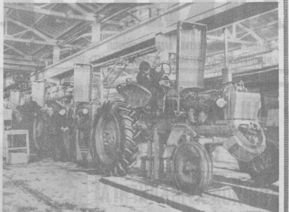
Суратда: тракторларни конвейер усулида йиғув цехи.
