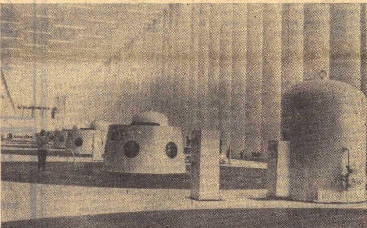
БИРЛАШГАН АРАБ РЕС-ПУБЛИКАСИ. Январ ойида Нил дарёсиданг Асвон гидро-энергетик комплексини қури-лиш тугалланди. Совет Итти-фонининг иқтисодий ва техника-вий ёрдами билан тикланган бу улкан иншоот араб ва со-вет халқлари дўстлигининг ра-зи бўлиб қолди. Суратда: ГЭСнинг машина зали.
