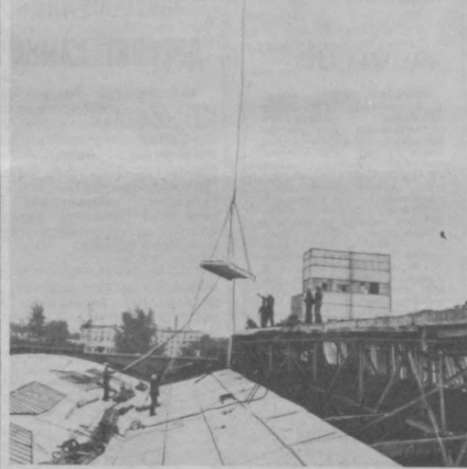
РОШКАР-ОЛА. За четыре дня вместо полутора месяцев проведена замена плит покрытый на производственном корпусе Марийского машиностроительного предприятия без остановки производства помоли ученые Марийского политехнического института имени А. М. Горького и летчики Куйбышевского авиационного училища гражданской авиации. Был разработан и осуществлен оптимальный вариант проведения монтажных работ с воздуха.
