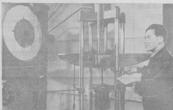
На Узбекском металлургическом заводе организована новая механическая лаборатория, которая дала возможность заводу сдавать протат по классу «А», идущий на ответственные конструкции. На снимке: техник комсомолец Эрин Баиев за испытанием образцов проката периодического профиля на разрыв.
