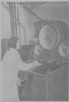
В центральной заводской лаборатории андийского завода «Строммашина» установлена новая универсальная разрывная машина для испытаний различных материалов на прочность. На снимке: начальник центральной заводской лаборатории А. К. Тюрина ведет работы по определению прочности материалов на новой машине. Фото С. Безносова.
