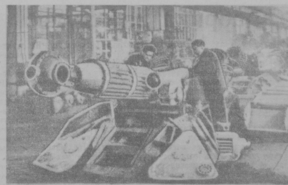
Венгерская Народная Республика. Завод «Красная звезда» изготовляет опытный образец нового угольного комбайна «Ф-5». Его можно использовать в штреках высотой 120 сантиметров. Новый проходческий комбайн имеет 4 режущих головки. Угольный комбайн «Ф-5» будет представлен на Всемирной выставке в Брюсселе. На снимке: новый комбайн в теще завода «Красная звезда».
