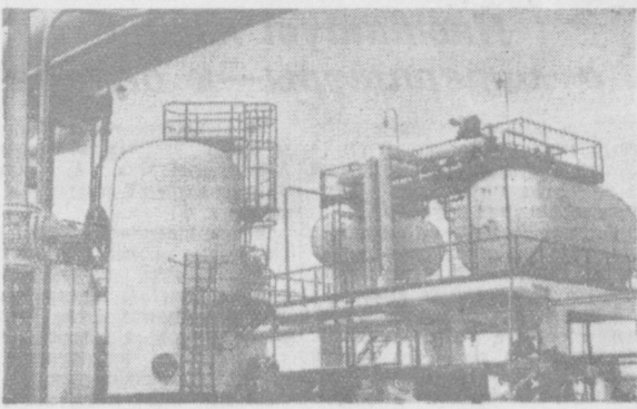
На строительстве Ферганского нефтеперерабатывающего завода к концу второго квартала 1958 года будет сдана в эксплуатацию электрообессоливающая установка. На снимке: общий вид электрообессоливающей установки. Фото И. Глауберсона.
