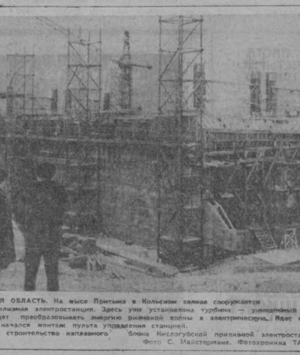
МУРМАНСКАЯ ОБЛАСТЬ. На мысе Притына в Кольском заливе сооружается Кисловская приливная электростанция. Здесь уже установлена турбина — крупнейший агрегат, который будет преобразовывать энергию приливной волны в электрическую. Идет строительство блока, начался монтаж пульта управления станции. НА СНИМКЕ: строительство наплавного блока Нисловской приливной электростанции. Фото С. Майстермана. Фотохроника ТАСС.
