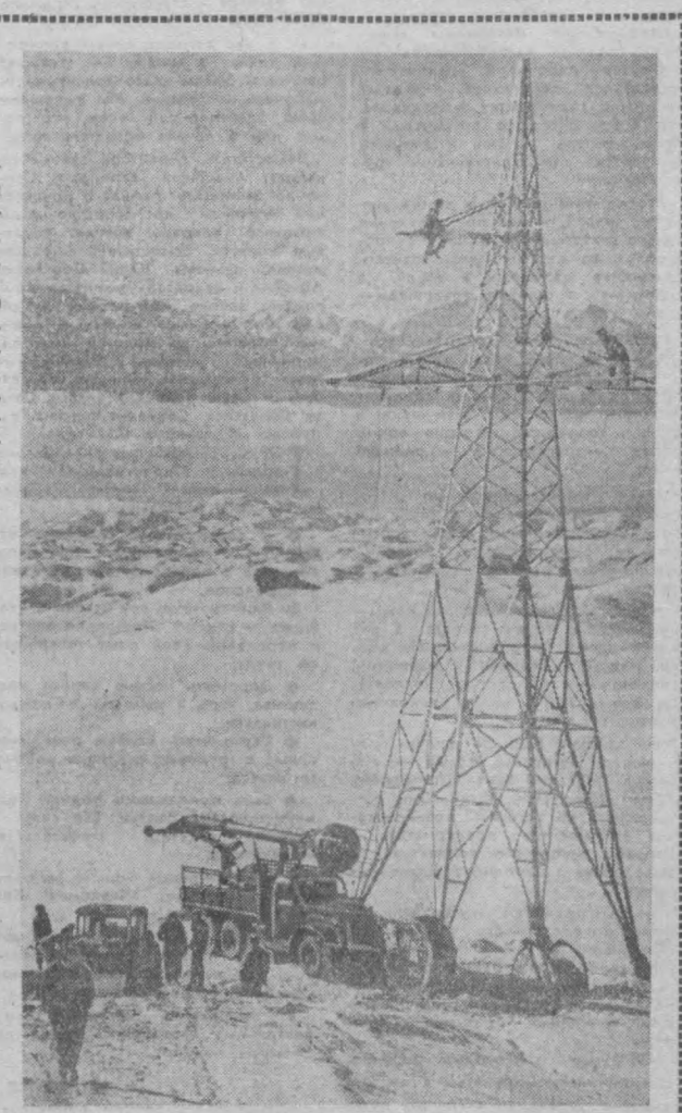
На снимке: ЛЭП в горах.
