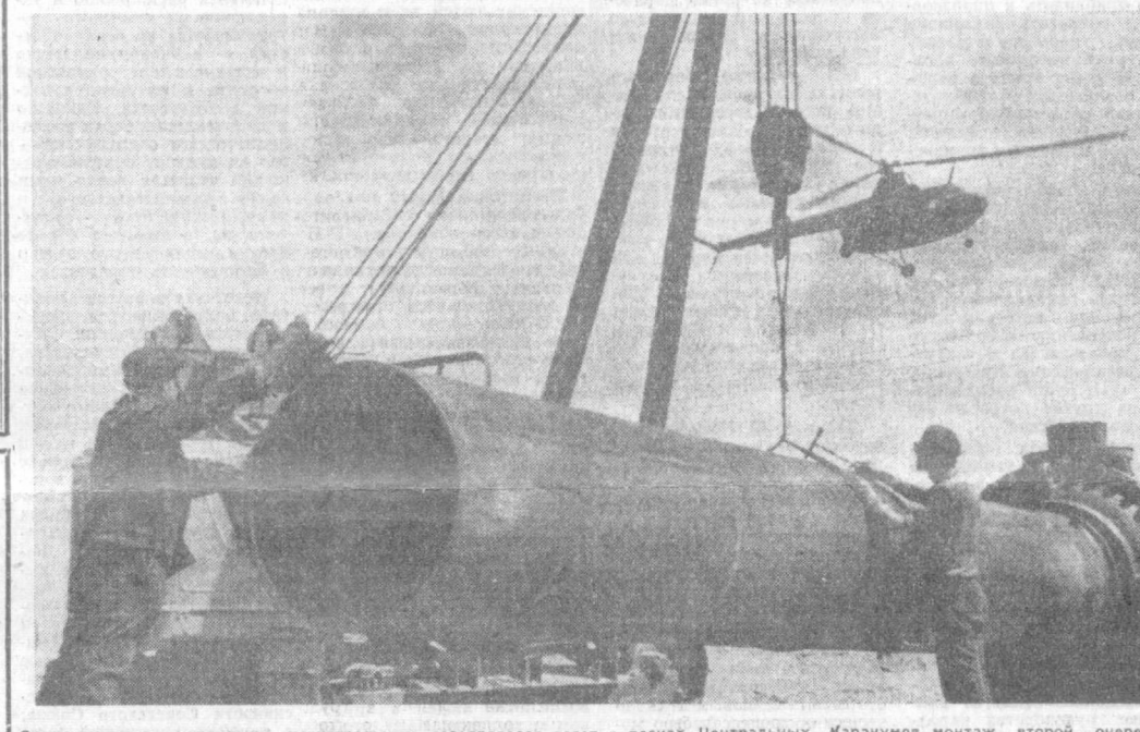
Среднеазиатское управление магистральных газопроводов ведет в лесках Центральных Каракумов монтаж второй очереди компрессорной станции № 1. Это — одно из звеньев большой работы по увеличению пропускной способности трубопровода, идущего в центральные районы страны. На снимке: один из участков строительства. Фото Р. ДЖУМАННАЗОВА.
