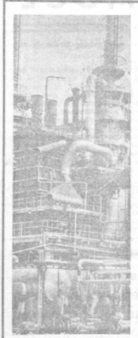
Чек зацвела — первое звено технологической линии по производству органики на Мавайском хлопководстве. Сейчас здесь ведется наладка контрольно-измерительных приборов и узлов автоматики. На снимке: один из участков чека зацвела.
