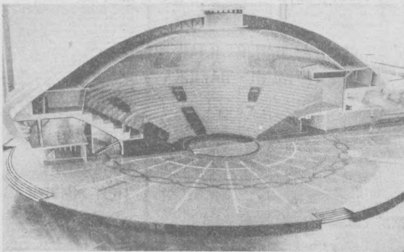
Манет Ташкентского цирка на 3000 посадочных мест. Он будет построен в районе улицы Хамзы.
