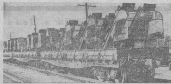
НА СНИМКЕ: новые машины для хлопковых заводов страны, отправленные заводом «Узхлопмаш».
