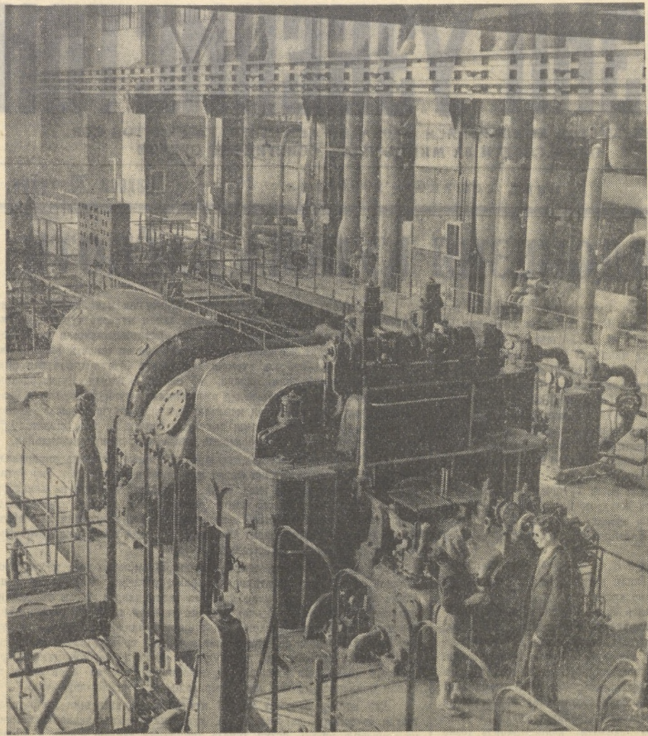
Рағли металлургия маркази — Омалик шаҳрида иссиқлик электростанциясининг биринчи наба. Ти ишта туширилади. Бу ТЭЦ ўрта Осиё энергетика системасига таъминланади. СУРАТДА: электростанциянинг турбина бўлими, Г. ПУН ФОТОС.
