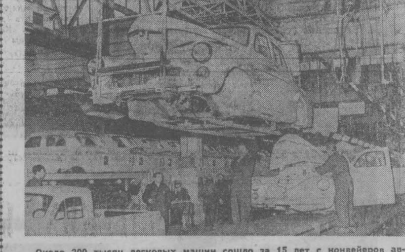
Около 200 тысяч легковых машин сошло за 15 лет с конвейера автомобильного завода «Варшава» в польской столице. Это предприятие, как и многие другие в Народной Польше, выросло на пустом месте. Построенный по советской лицензии, благодаря советской помощи, Варшавский автозавод уверенно идет вперед, разрабатывая новые марки машин, увеличивая свою производственную мощность. Фото ЦАФ—ТАСС.
