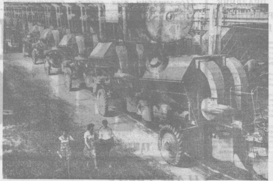
Ежедневно десятки голубых кораблей «ХТ-1,2» сходят с конвейера главного сборочного цеха завода «Ташсельмаш».
