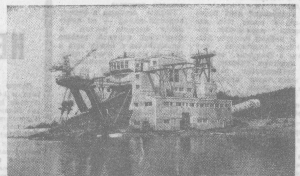
На Урале, в золотонной долине реки Миасс, вступила в строй действующая новая драга — плавучее землерезательное сооружение, при помощи которого разрабатывают россыпные месторождения золота. Все процессы работы на этом горнодобывающем агрегате полностью механизированы. НА СНИМКЕ: новая драга. Фото В. Каушанова. (АПН).
