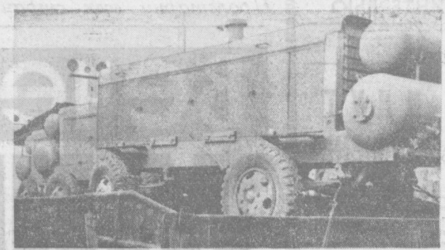
ЕЩЕ ОДИН НОВЫЙ АГРЕГАТ СОБРАН В СБОРОЧНОМ ЦЕХЕ ЗАВОДА «КОМПРЕССОР» И ПОДГОТОВЛЕН К ОТПРАВКЕ.
