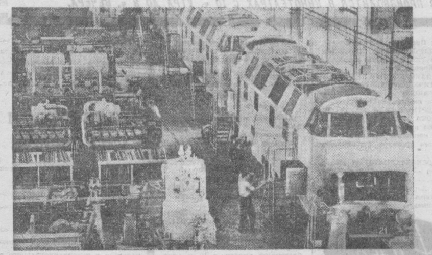
НА СНИМКЕ: народное предприятие имени Карла Маркса в Потсдаме. Здесь строятся мощные гидроэлектрические тепловозы.
