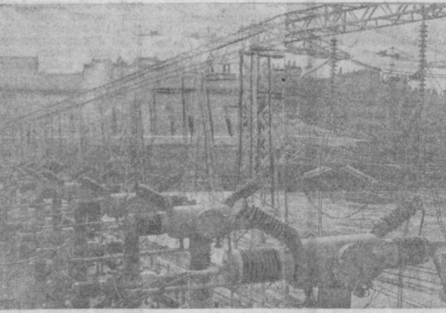
Строители Красноярской ГЭС закончили монтаж четвертого агрегата. Идут последние пригонки и его испытание на холостых оборотах. К 50-летию юбилею Ленинского комсомола агрегат намерено сдать в эксплуатацию. НА СНИМКЕ: открытое распределительное устройство Красноярской ГЭС готово принять ток четвертого агрегата. Фото Л. Портера. (Фотокроника ТАСС).
