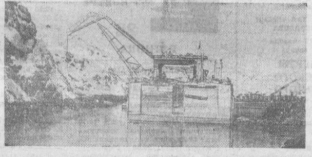
МУРМАНСКАЯ ОБЛАСТЬ. На побережье Баренцева моря в губе Кислой Севгидрострой заканчивает сооружение опытной приливной электростанции. НА СНИМКЕ: здание ПЭС. На нем монтируется кран для подъема затворов турбины. Фото Л. Бернштейна.
