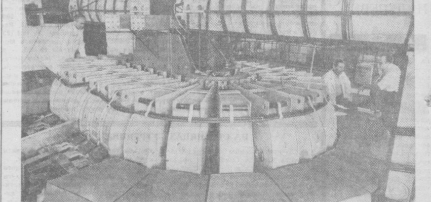
НА СНИМКЕ: термоядерная установка «Ураган-1» — один из крупнейших в мире стеллараторов. Здесь изучаются вопросы удержания высокотемпературной плазмы в зависимости от параметров плазмы и магнитной системы установки. Установку научный сотрудник А. Г. Диний, кандидат физико-математических наук В. А. Супруненко, доктор физико-математических наук В. Т. Толок. Фото А. Татаренко. (Фотохроника ТАСС).
