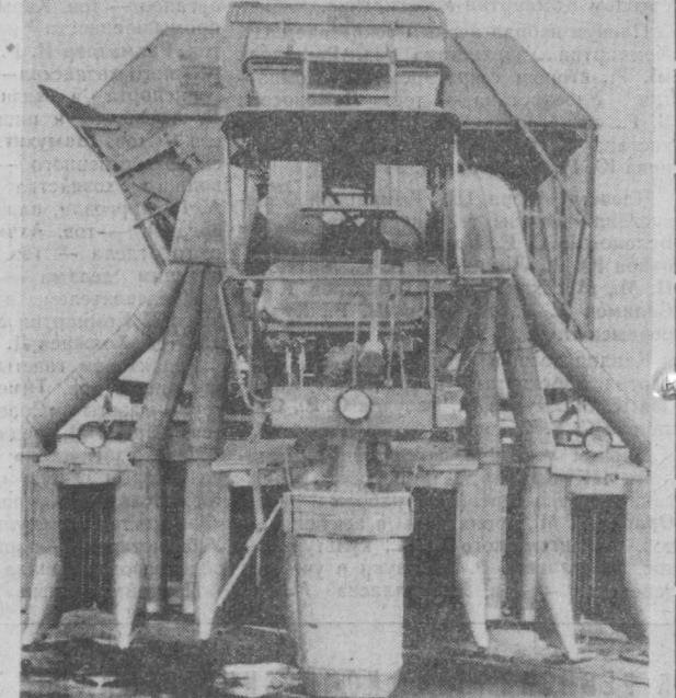
НА СНИМКЕ: машина «ХН-3,6». Фото И. Кокорева.
